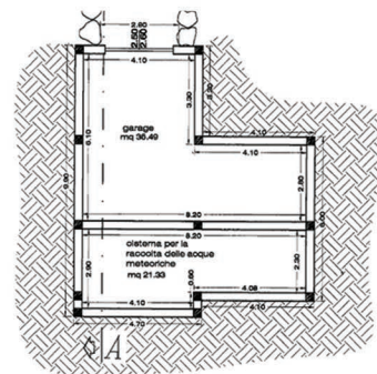
pianta piano seminterrato
